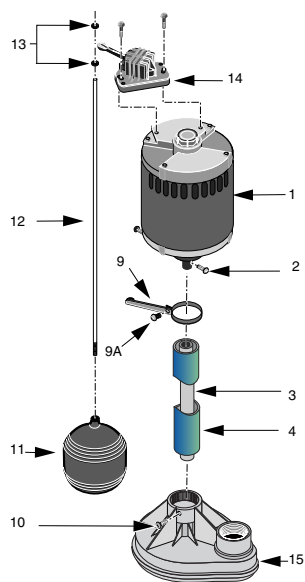
Modèle FPPM3600D-08
