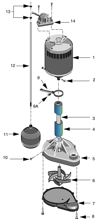
Modèle FPPSS3000-08
