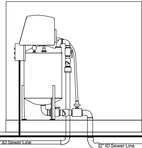
2. Edson VacuMaster
