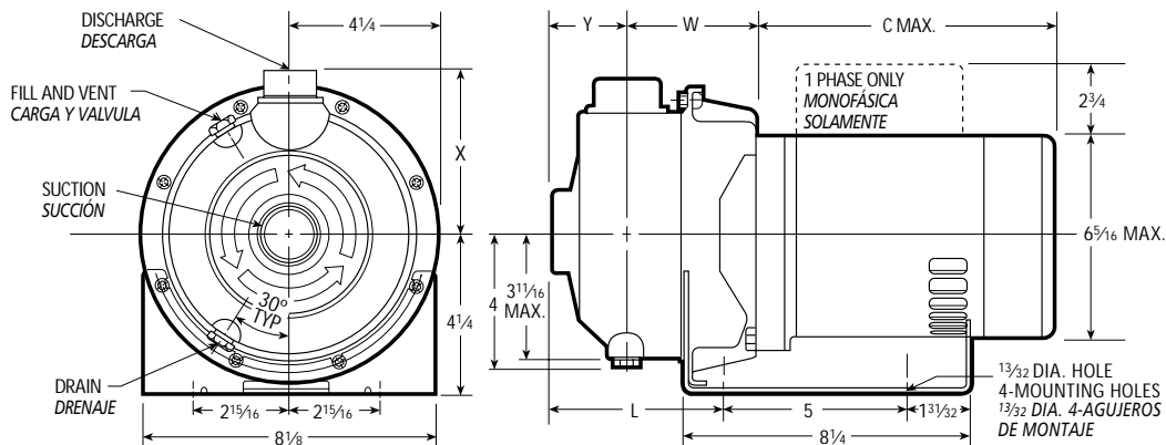
ODP and TEFC 1\frac{1}{2} , 2 and 3 HP, ODP y TEFC 1\frac{1}{2} , 2 y 3 HP
