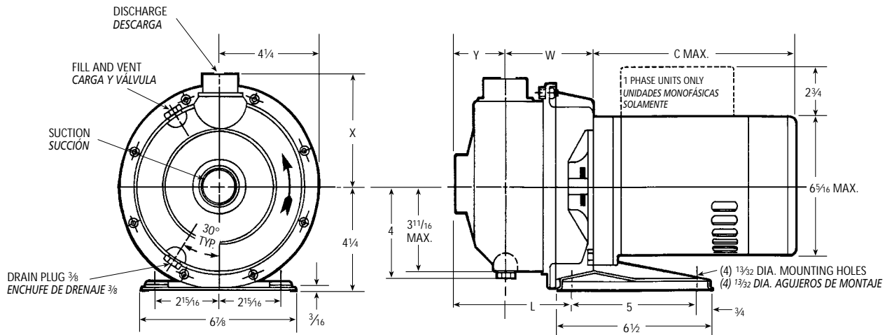
ODP and TEFC \frac{1}{2} , \frac{3}{4} and 1 HP, ODP y TEFC \frac{1}{2} , \frac{3}{4} y 1 HP
