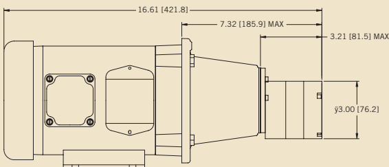
56C NEMA 0.5 HP MOTOR
