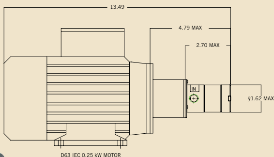
D63 IEC 0.25 kW MOTOR
